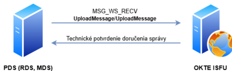
Obrázok 2 Rozhranie MSG_WS_RECV
