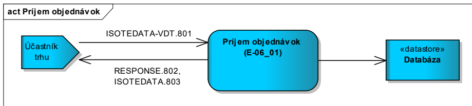
Obrázok 24 Schéma prijmu objednávky ÚT
