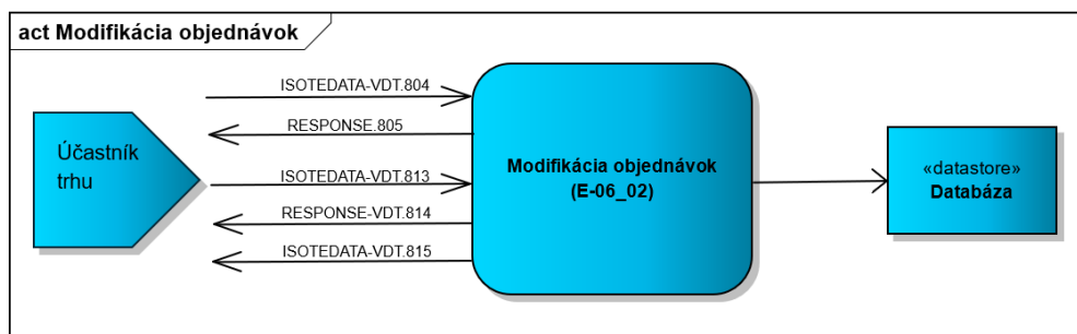
Obrázok 25 Schéma modifikácie objednávky ÚT
