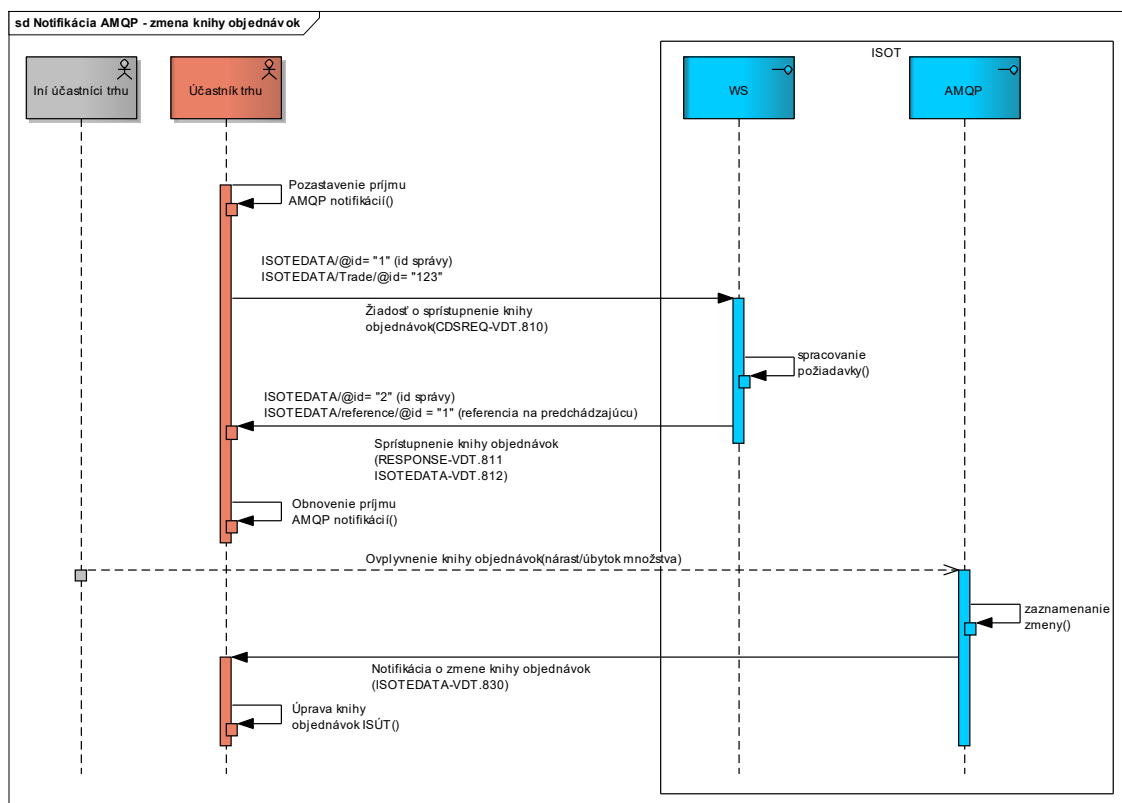
Obrázok 44 Schéma následnosti posielaných správ – zmena knihy objednávok (AMQP notifikácia)
